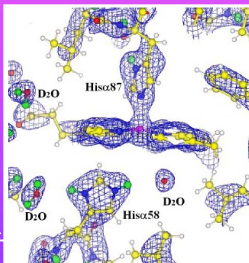
ヒト血液ヘモグロビン分子内で見られた重水素原子（緑で表示）と核密度分布（フーリエ）図
