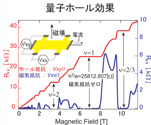
2 層系 \nu = 1 量子ホール状態
