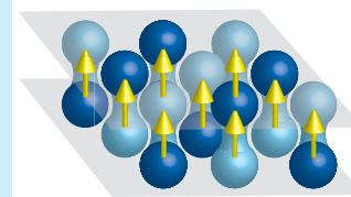
2 層系 \nu = 1 量子ホール状態
