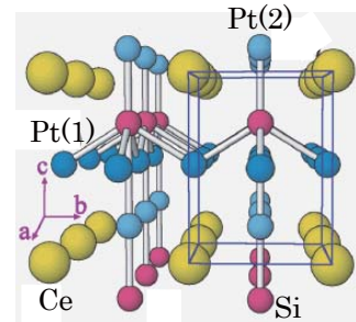
超伝導体 \text{CePt}_3\text{Si} の結晶構造
