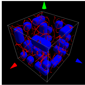
図4. 二相状態の合金を変形すると界面から柔らかい領域にひも状の欠陥ができる。
