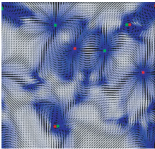
図1. 液晶中のイオン。 僅かでも強相関状態にある。
