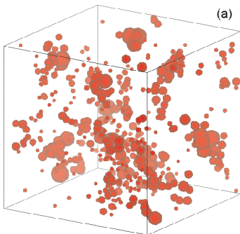
図3. ガラスの動的不均一性。低温では可動領域と不可動領域が不均一に混在。
